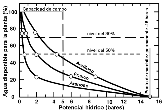
Figura 1. Diagrama con curvas características del contenido de humedad y tensión para suelos arenosos, arcillosos y francos. Tomada del Manual de Ingeniería Nacional (EU), 210-VI.
